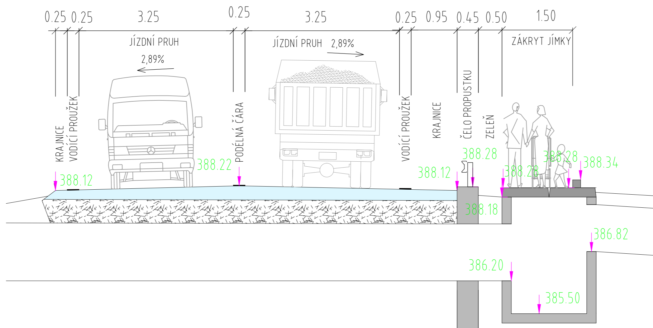
PŘÍČNÝ ŘEZ I - I 1:50
