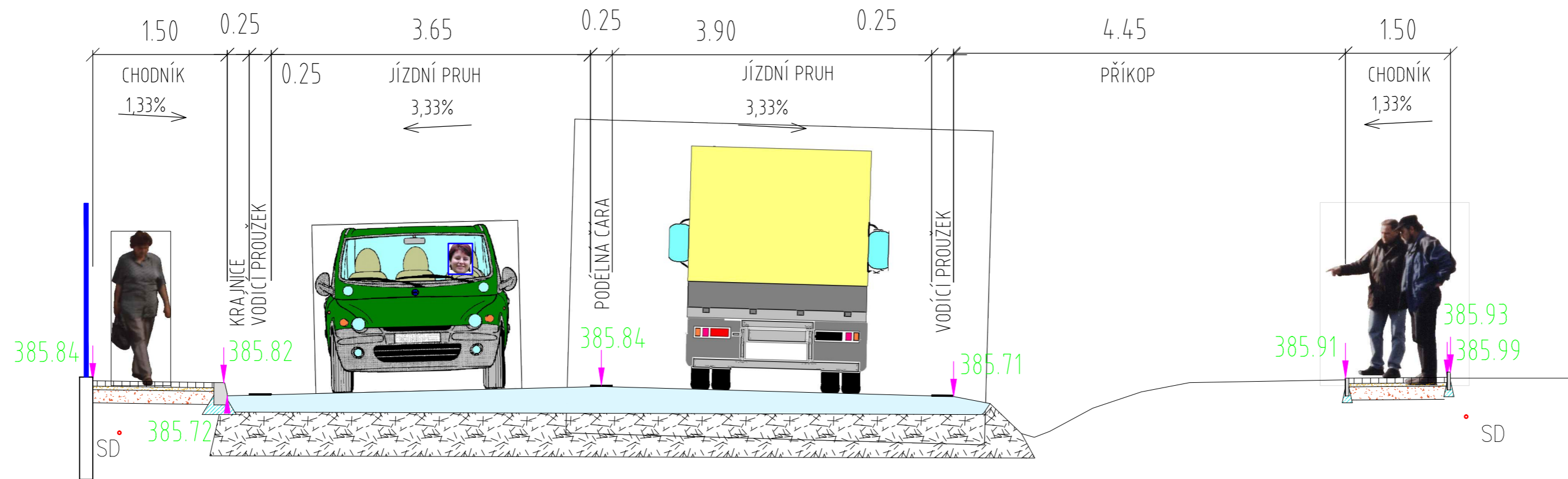
PŘÍČNÝ ŘEZ G - G 1:50
