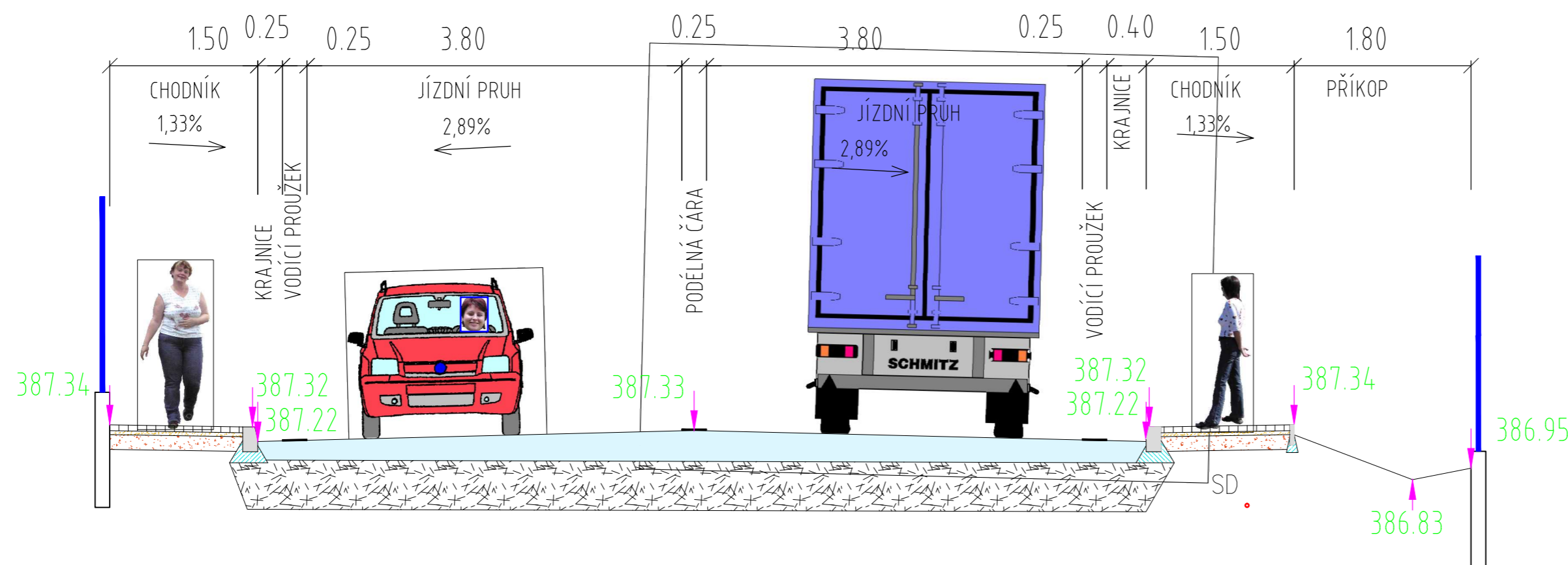
PŘÍČNÝ ŘEZ H - H 1:50
